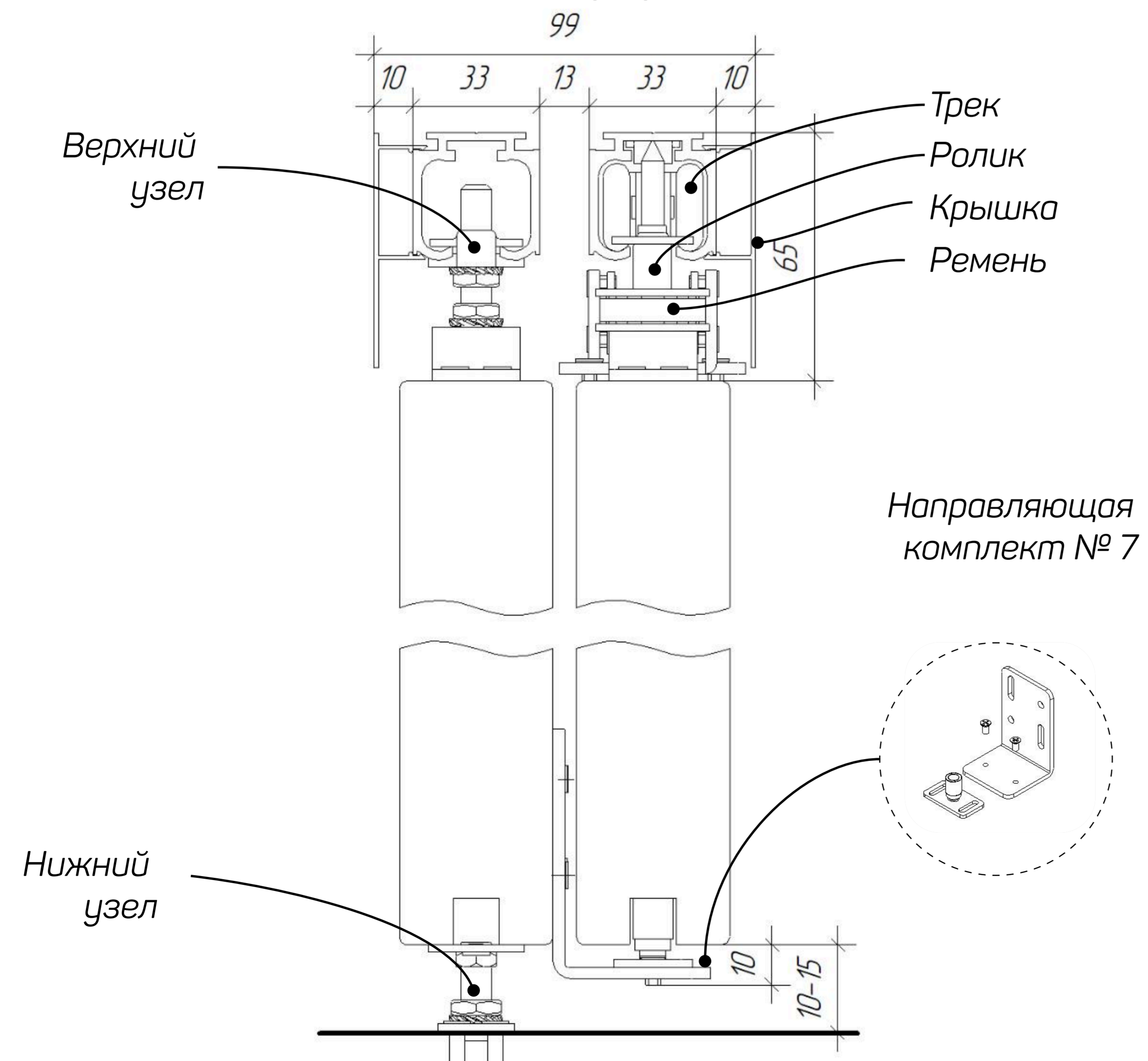
ВЕРТИКАЛЬНОЕ СЕЧЕНИЕ
